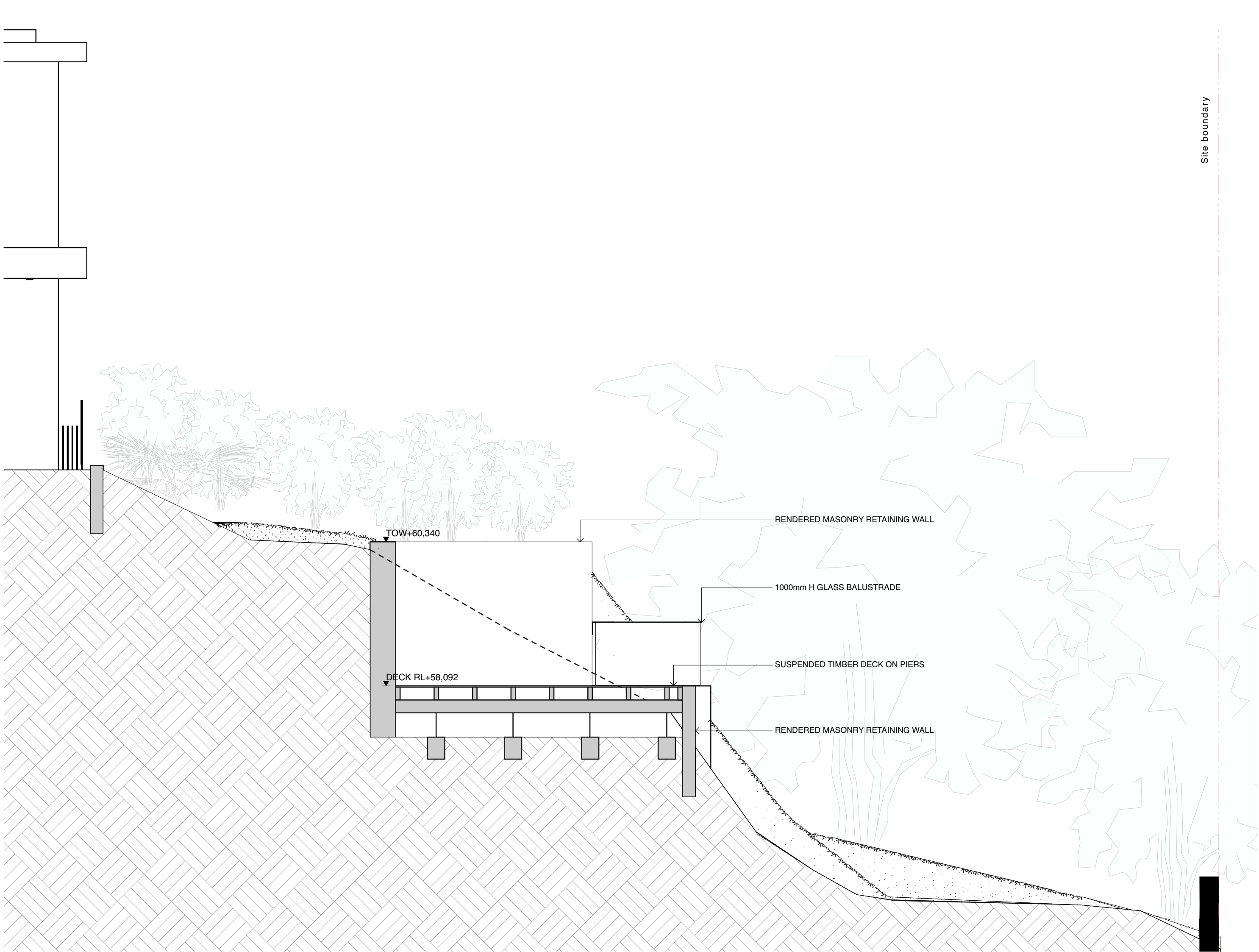
Section F/F
